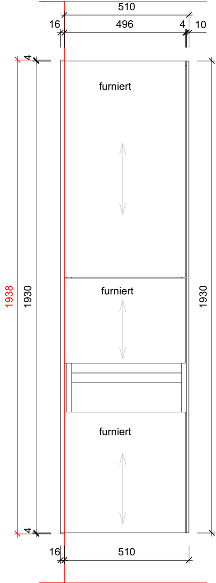
Ansicht 2
